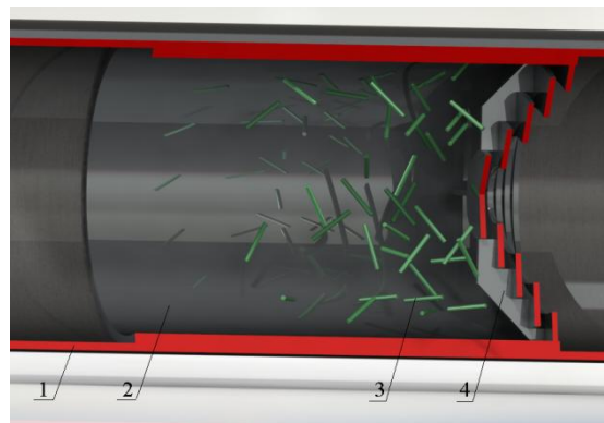
Fig. 21. Labyrinth
