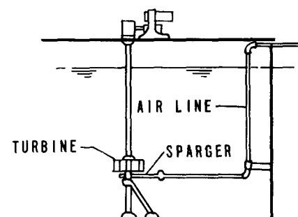
B-3 AGITATOR SPARGED-SYSTEM
