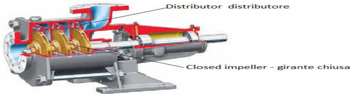
horizontal multistage pump pompa orizzontale multistadio
