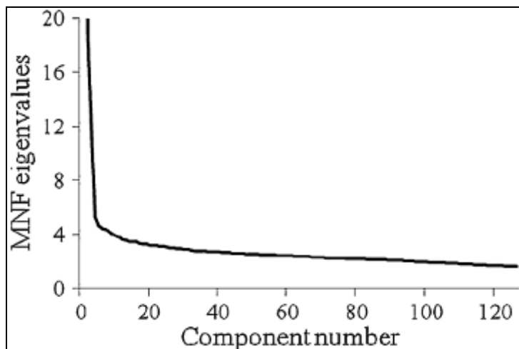
Fig. 10. MNF eigenvalues variation trend
